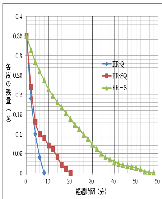
図1 各液のシャーレ内の揮発減量グラフ
