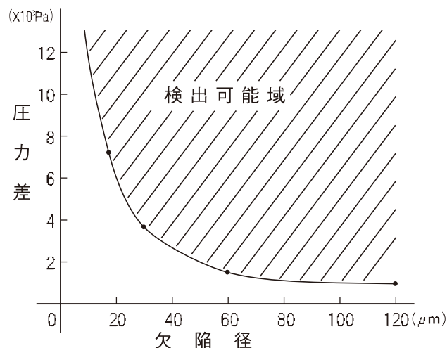
図1. 検出可能な孔径と圧力との関係
