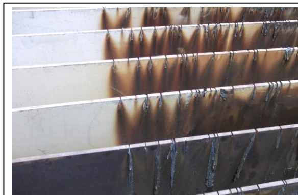
(上部:ドロスガード塗布部 下部:無塗布部) ※上部は、下部に比べ大幅にドロス付着が少ない。
