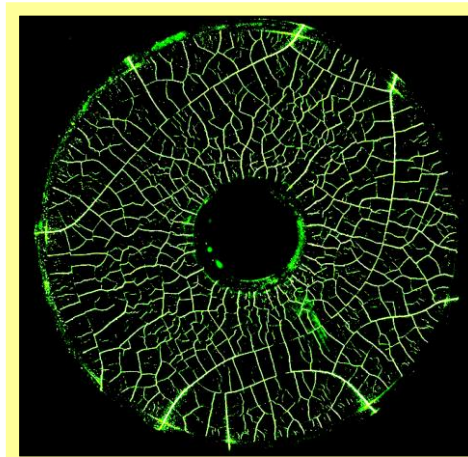
蛍光磁粉ジキチェックF-330の適用例.
